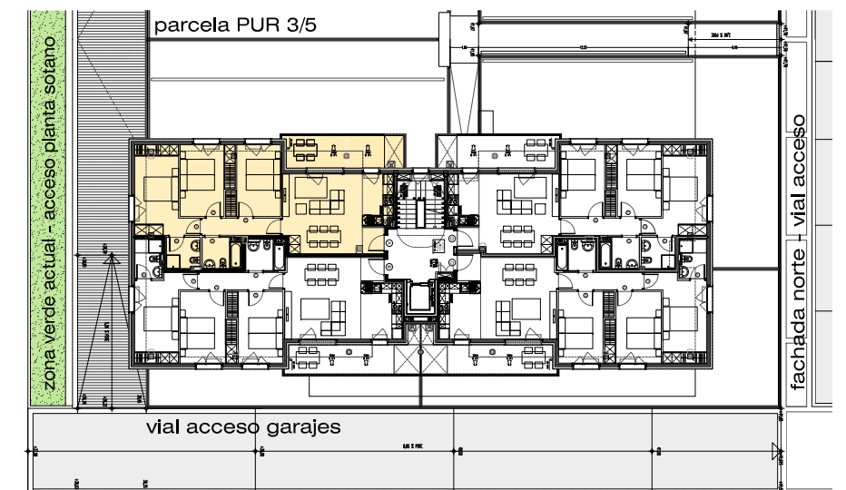
localizacion de la vivienda en planta
