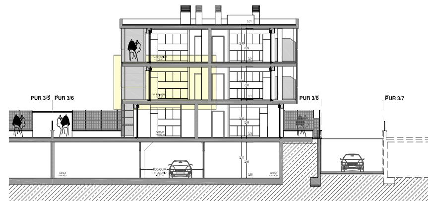
localizacion de la vivienda en seccion
